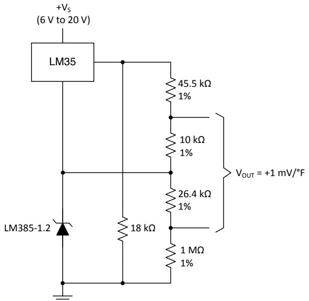
Figure 21. Fahrenheit Thermometer
